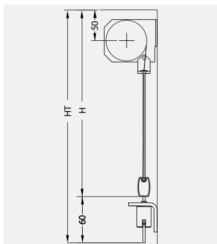
Guidage câbles
